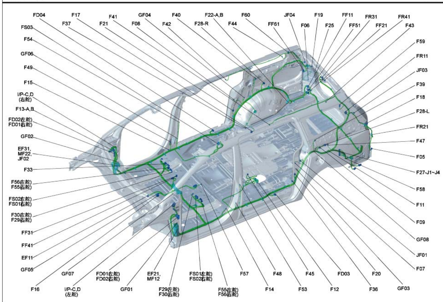
底板线束(1)
